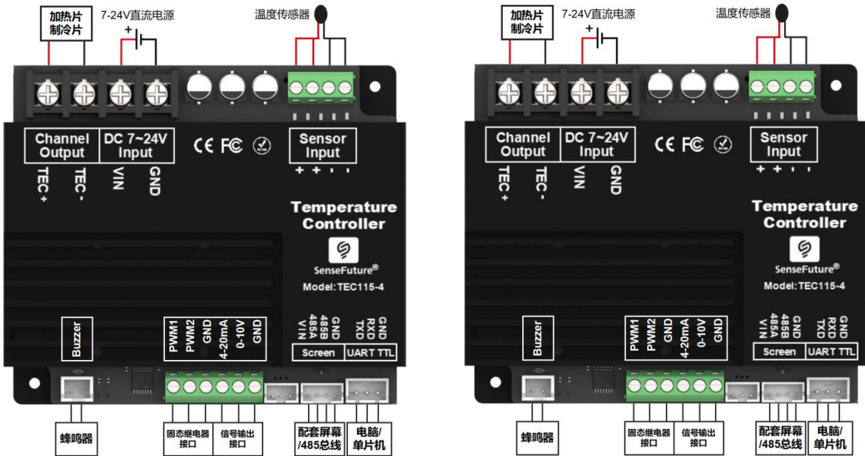
TEC107-4/115-4 系列温控器接线图 温控器引脚说明表
