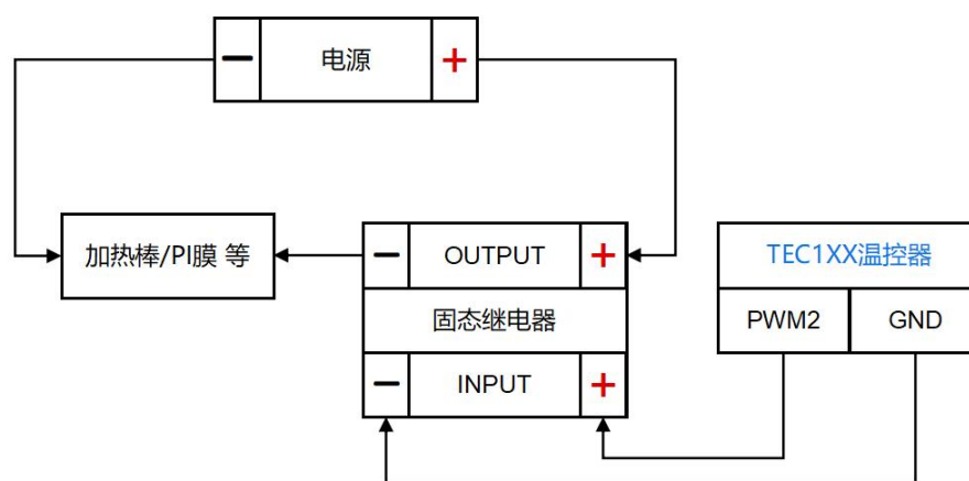
固态继电器单制冷（上图）制热（下图）接线方法图
