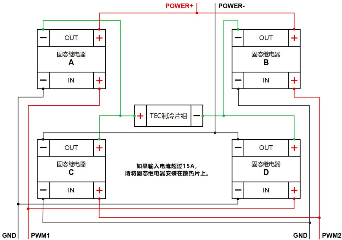
固态继电器接线方法图
