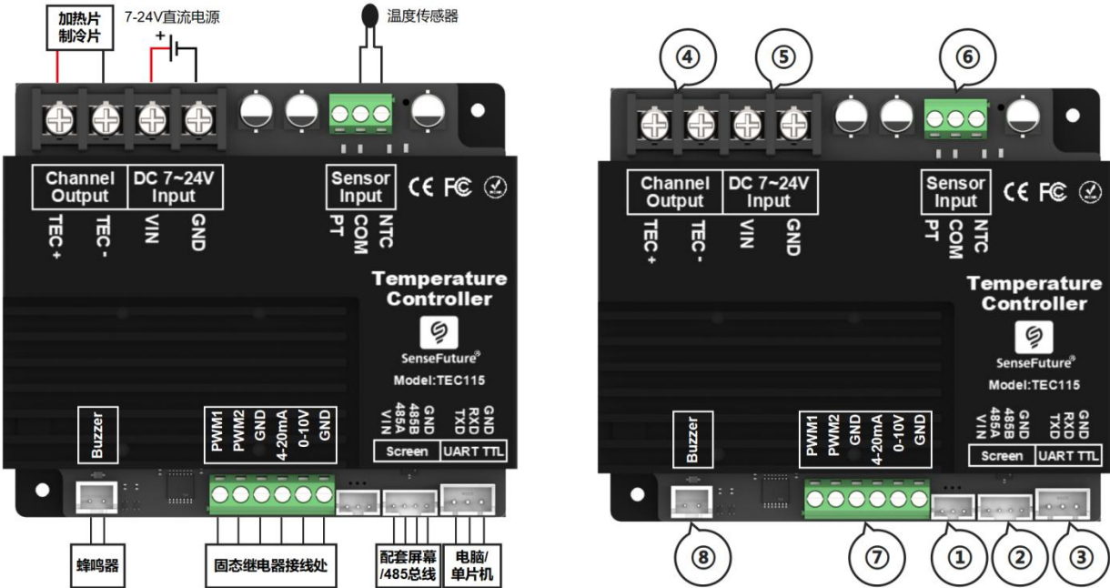
TEC107/115 系列温控器接线图
